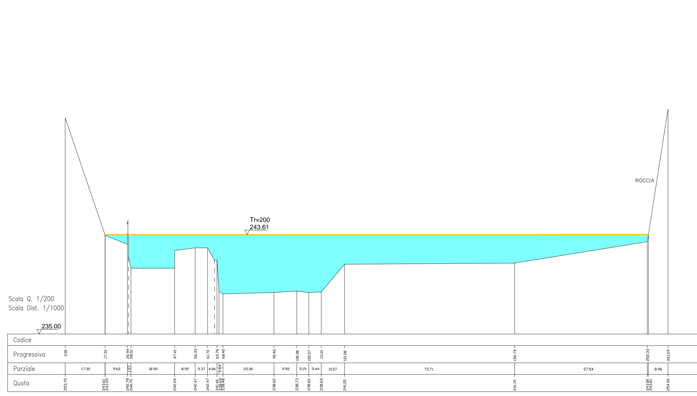
SEZIONE 39 Scale: 1:1000/200
