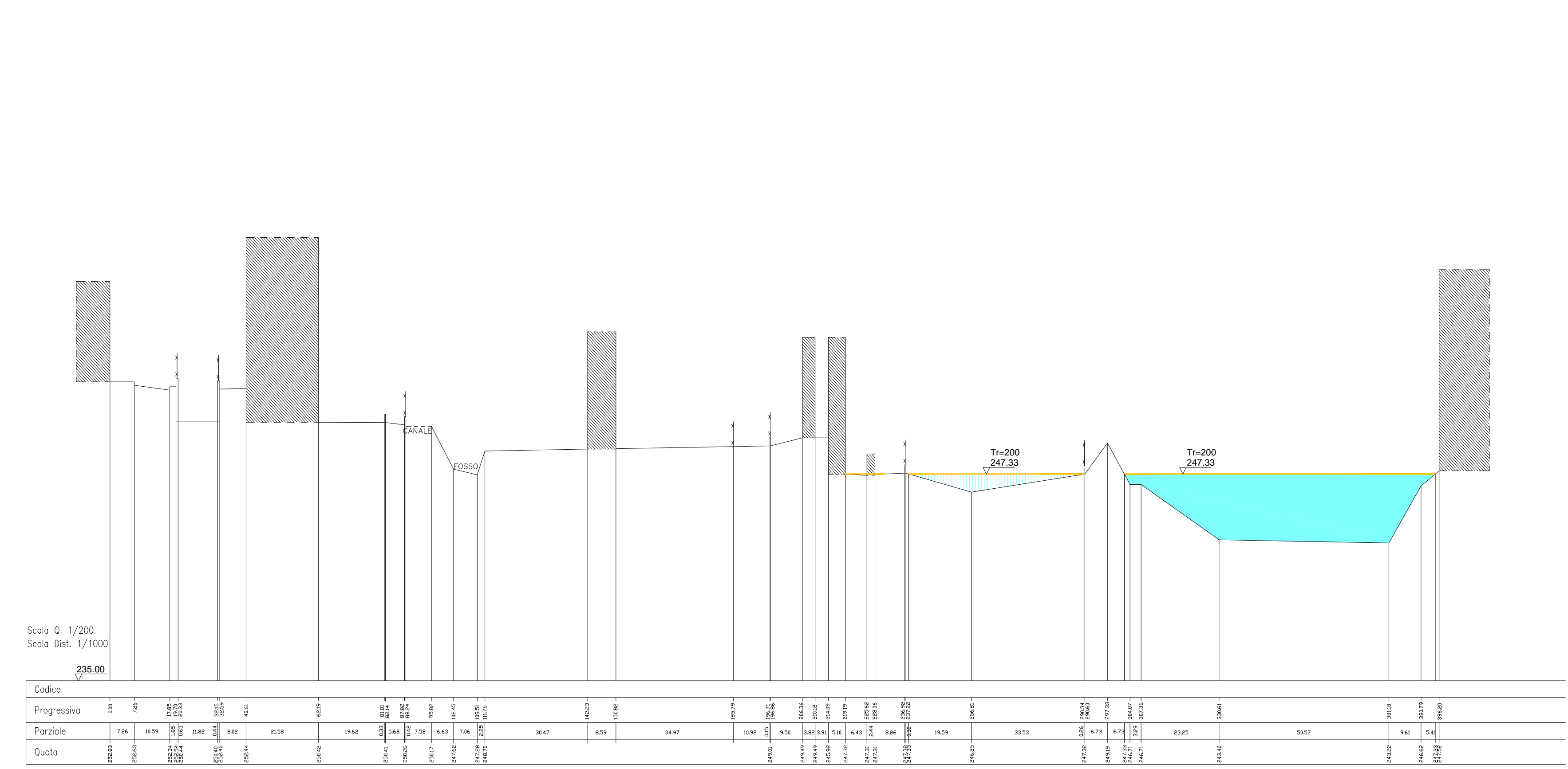
SEZIONE 41 Scale: 1:1000/200
