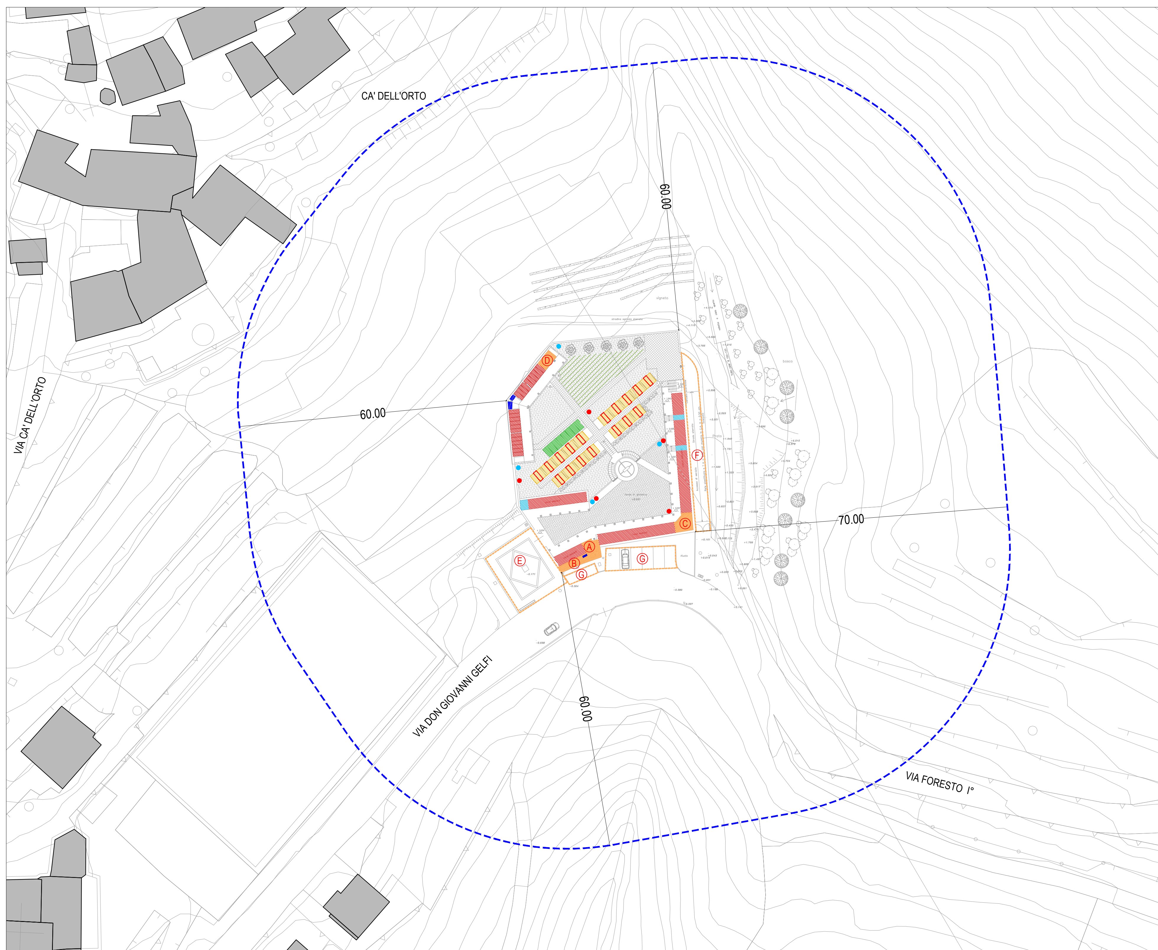
PLANIMETRIA GENERALE DELLO STATO DI FATTO scala 1:500
