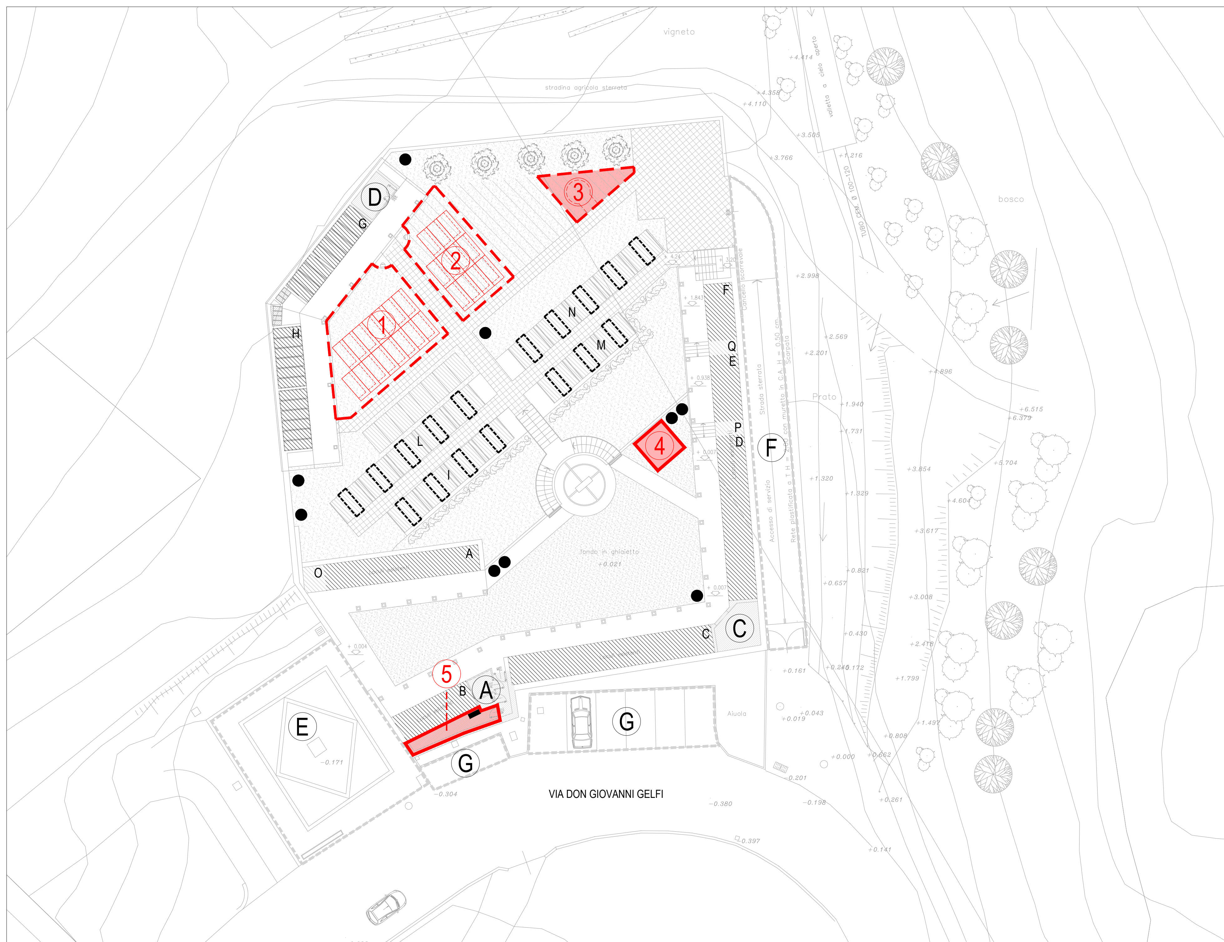
PLANIMETRIA GENERALE DI RAFFRONTO scala 1:200
