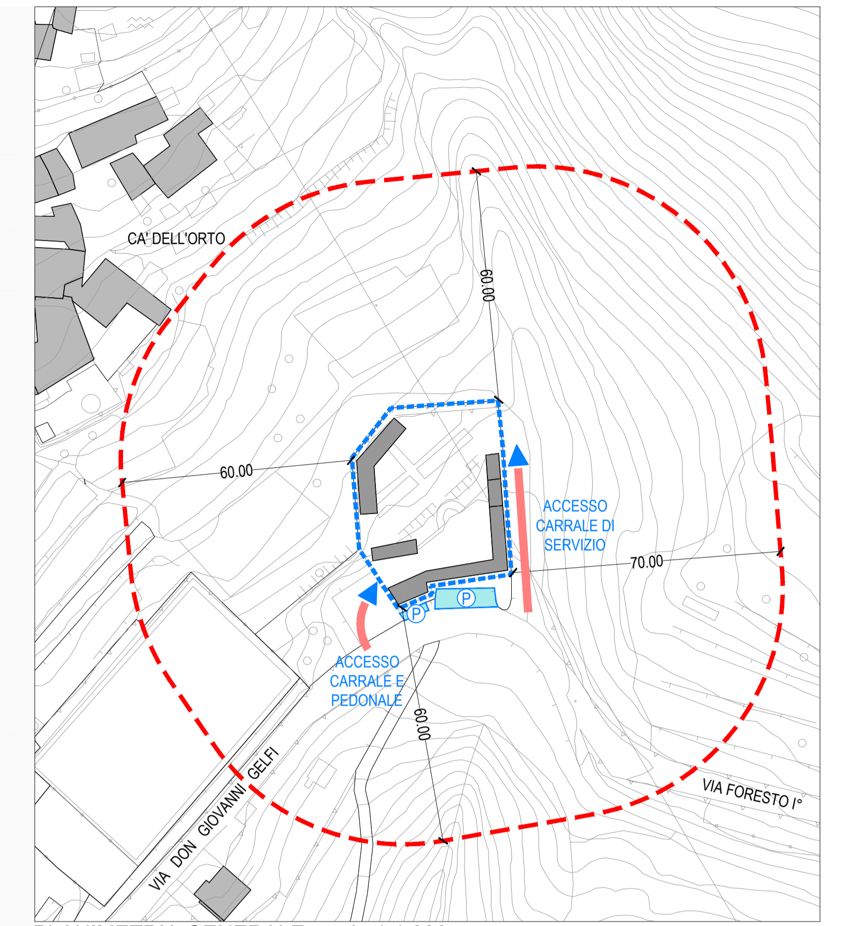
PLANIMETRIA GENERALE scala 1:1.000
