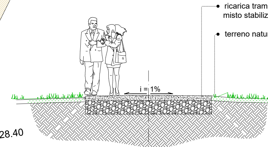
DETTAGLIO INTERVENTI SEZIONE D-D' Scala 1:50
