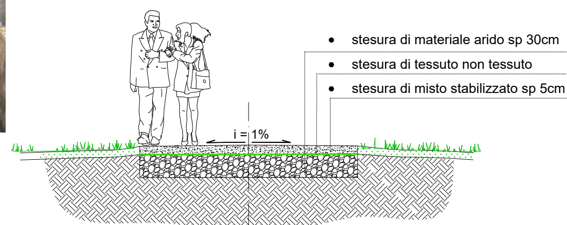
DETTAGLIO INTERVENTI SEZIONE B-B' Scala 1:50
