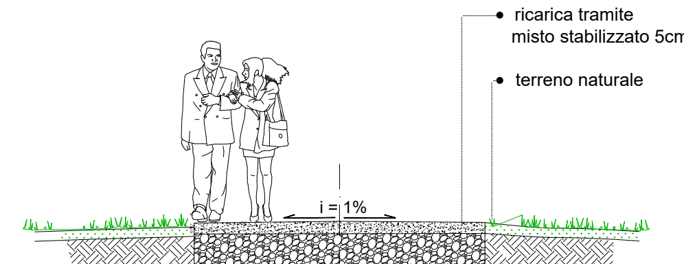
DETTAGLIO INTERVENTI SEZIONE C-C' Scala 1:50
