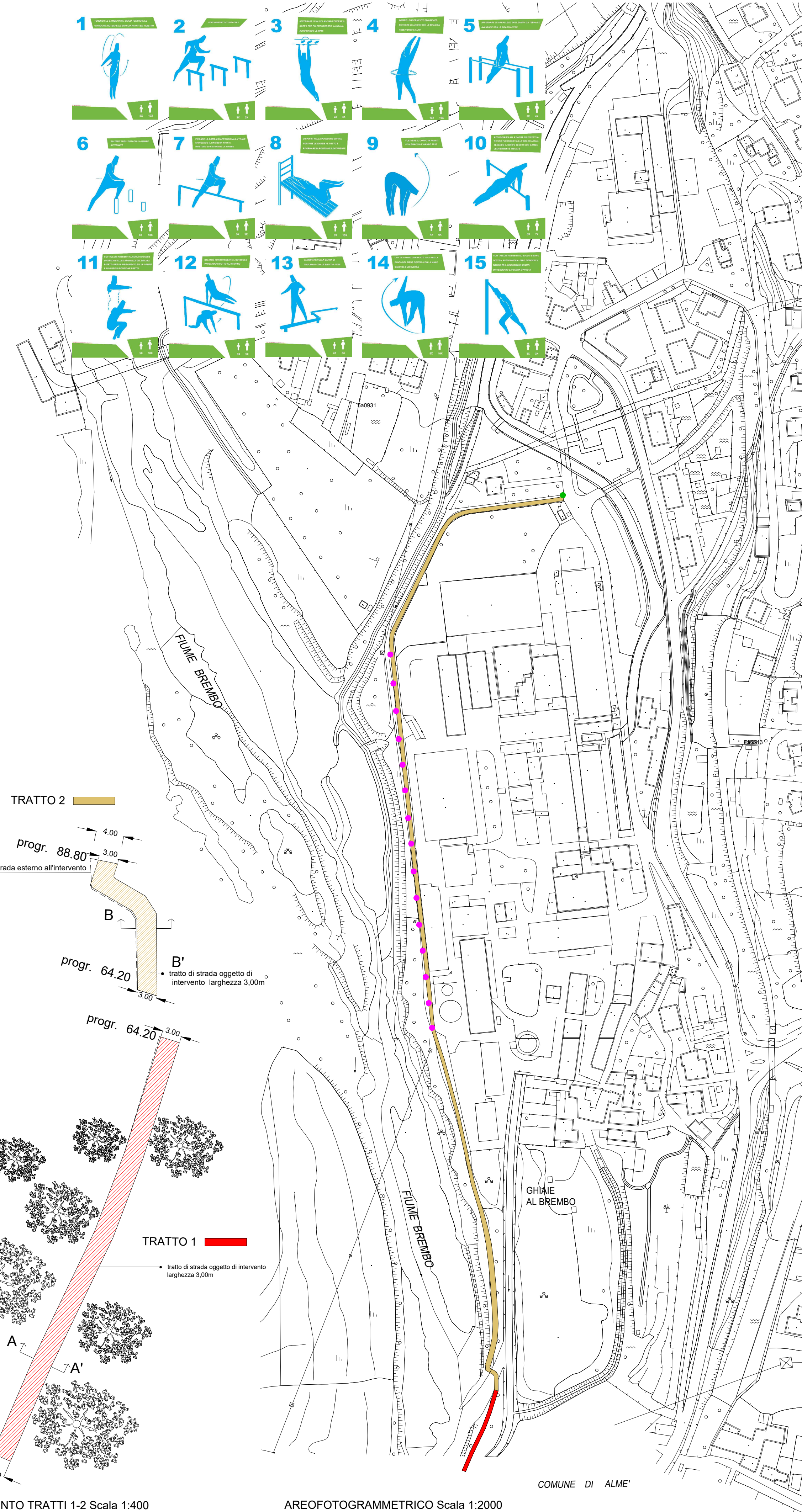
PLANIMETRIA D'INTERVENTO TRATTI 1-2 Scala 1:400
