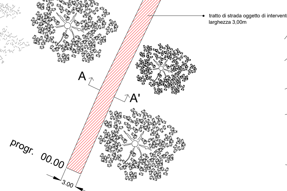
PLANIMETRIA D'INTERVENTO TRATTI 1-2 Scala 1:400
