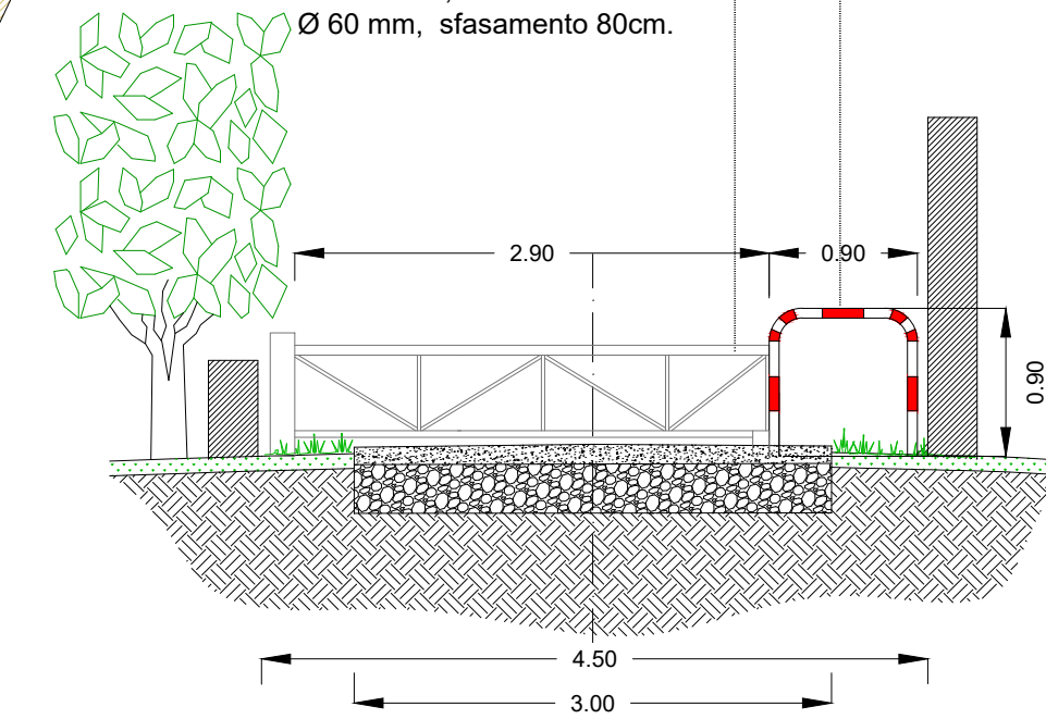
DETTAGLIO INTERVENTI SEZIONE D-D' Scala 1:50
