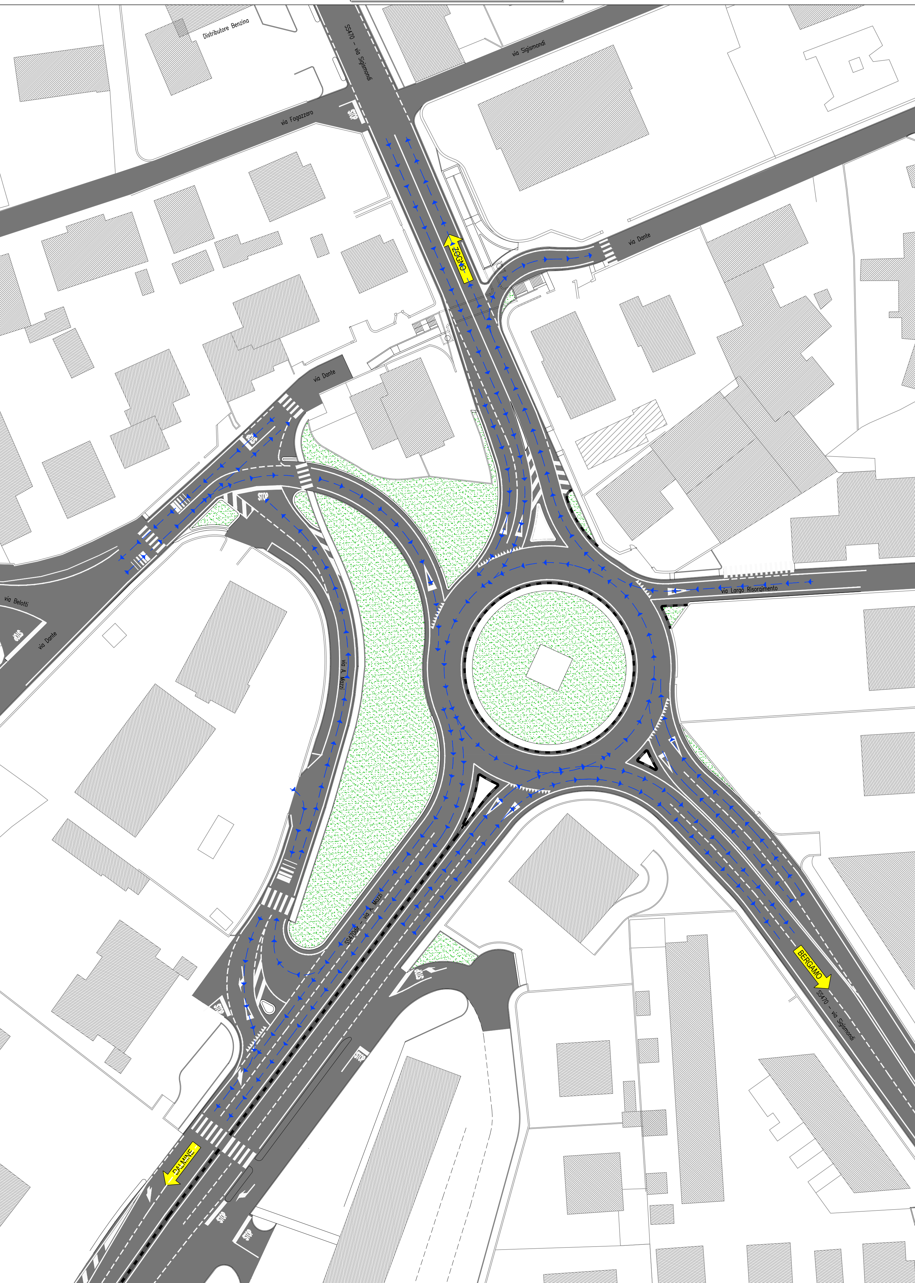
PLANIMETRIA GENERALE VIABILITA' ESISTENTE - scala 1:500
