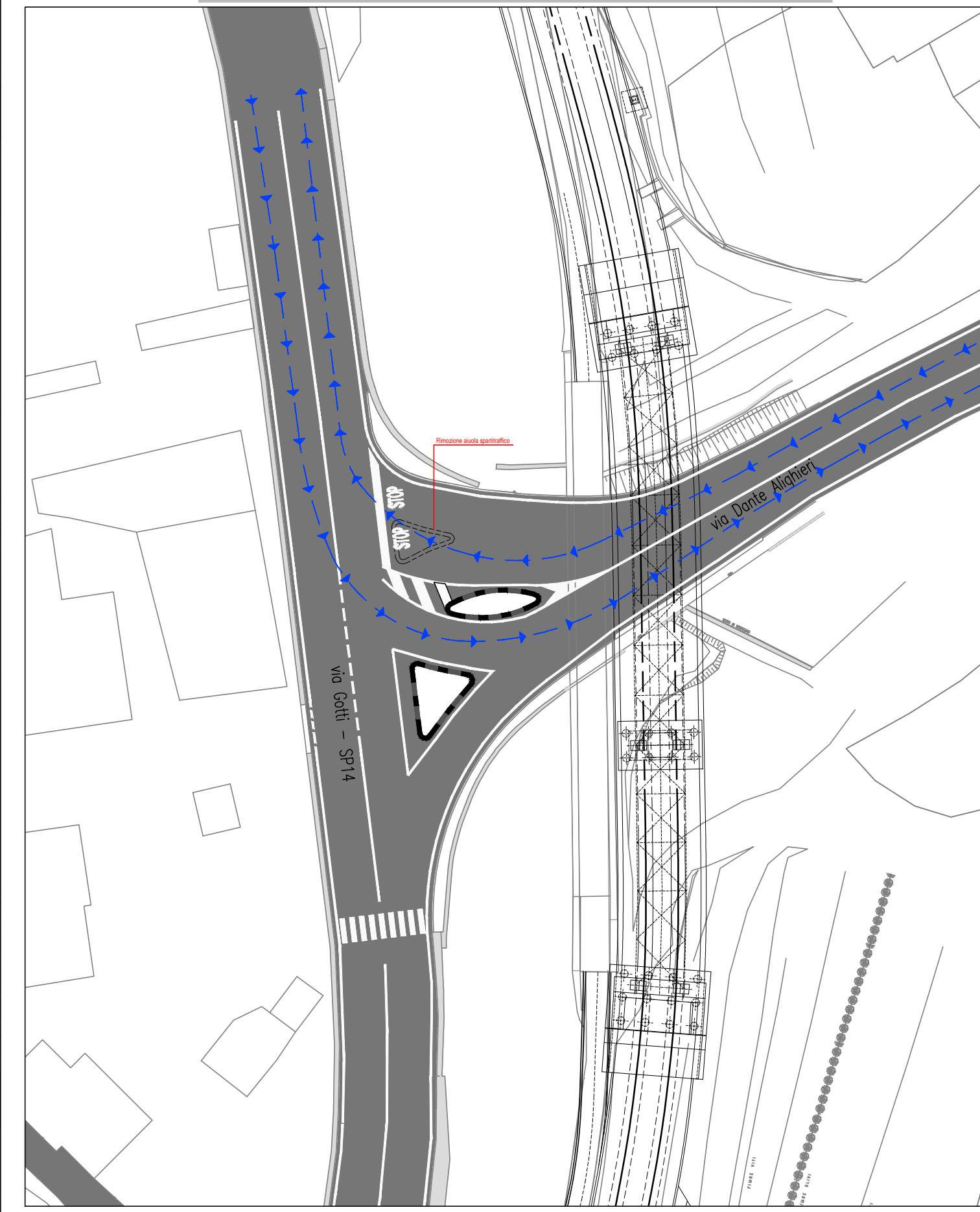
PLANIMETRIA INNESTO VIA DANTE/VIA GOTTI CON MODIFICA VIABILITA' - scala 1:500
