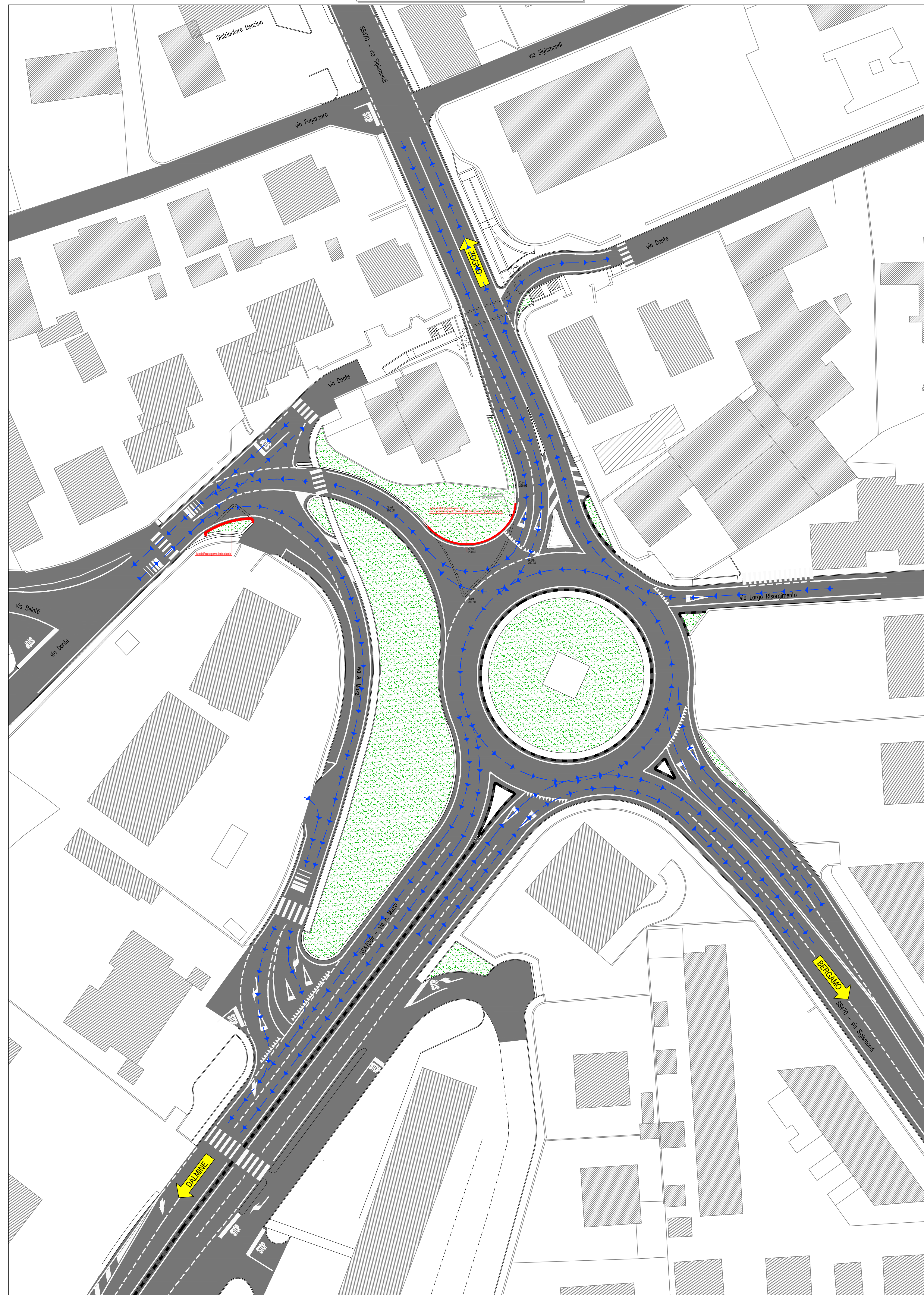
PLANIMETRIA GENERALE CON MODIFICA VIABILITA' - scala 1:500
